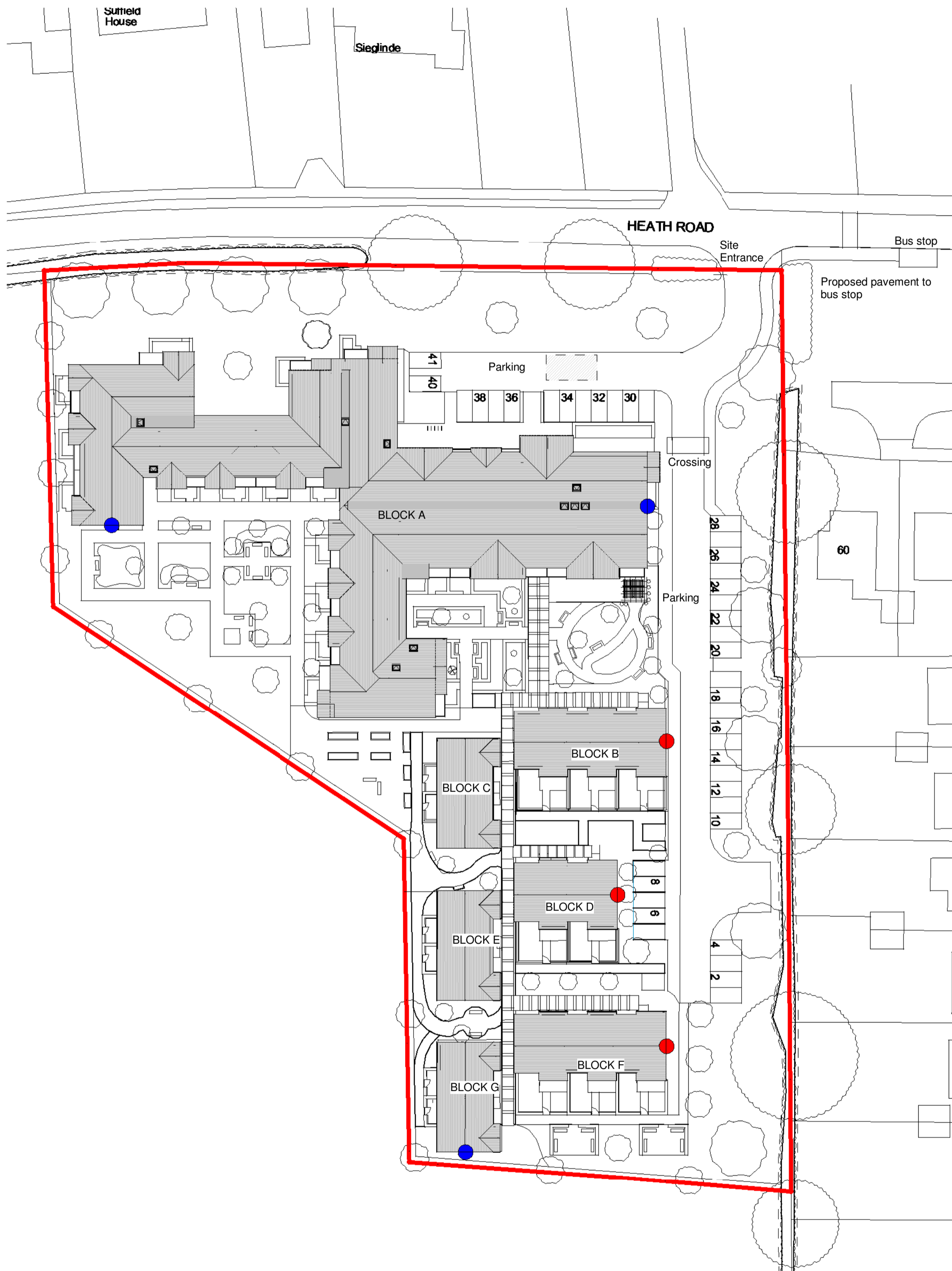
1 Block Plan 1 : 500
